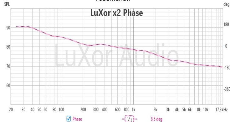
Fázismenet:
