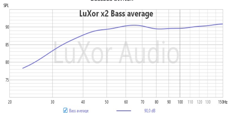
Basszus átvitel:
